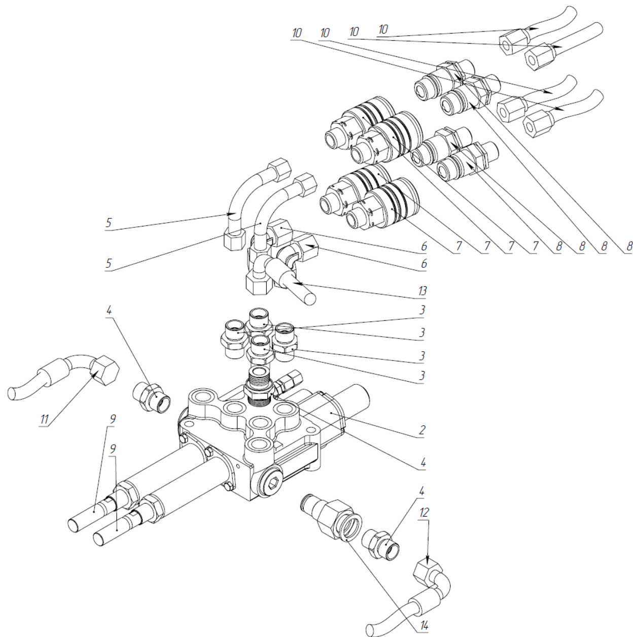
Опорная конструкция T229 к трактору МТЗ 1221 КАТАЛОГ ЗАПЧАСТЕЙ
